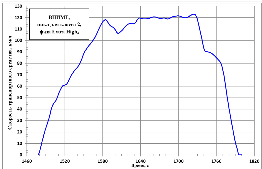
Рис. А1/6 ВЦИМГ, цикл для класса 2, фаза Extra High 2
