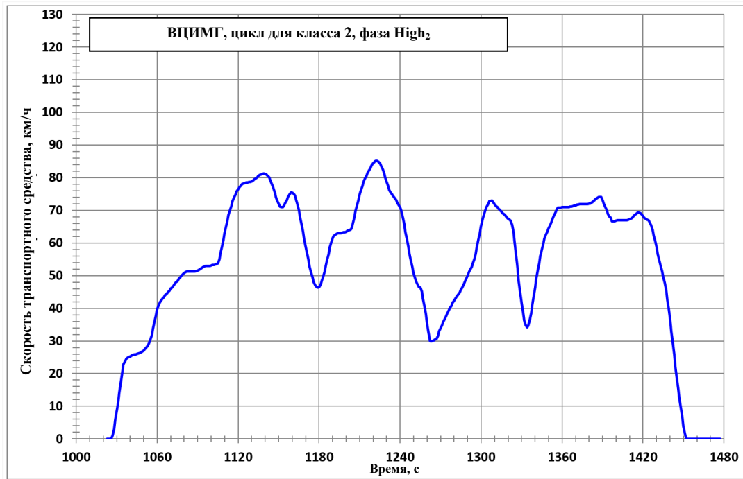
Рис. А1/5 ВЦИМГ, цикл для класса 2, фаза High 2
