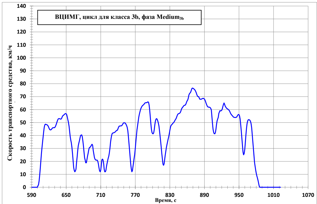
Рис. А1/9 ВЦИМГ, цикл для класса 3b, фаза Medium 3b
