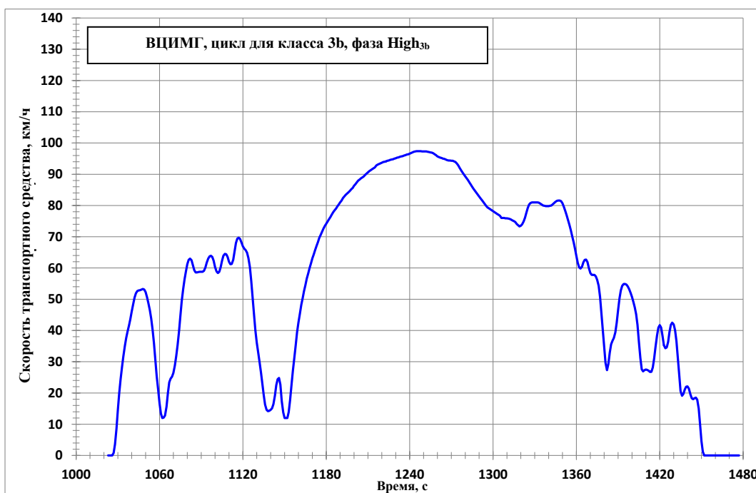
Рис. А1/11 ВЦИМГ, цикл для класса 3b, фаза High 3b
