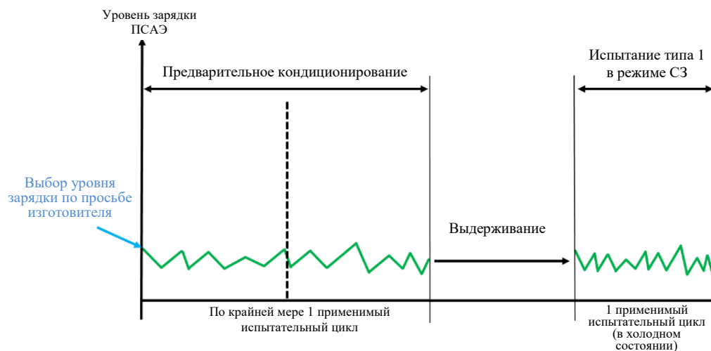
Рис. A8.App1/2 ГЭМ-ВЗУ, испытание типа 1 в режиме сохранения заряда
