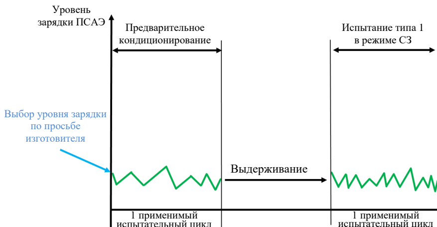
Рис. A8.App1/5 ГЭМ-БЗУ и ГТСТЭ-БЗУ, испытание типа 1 в режиме сохранения заряда
