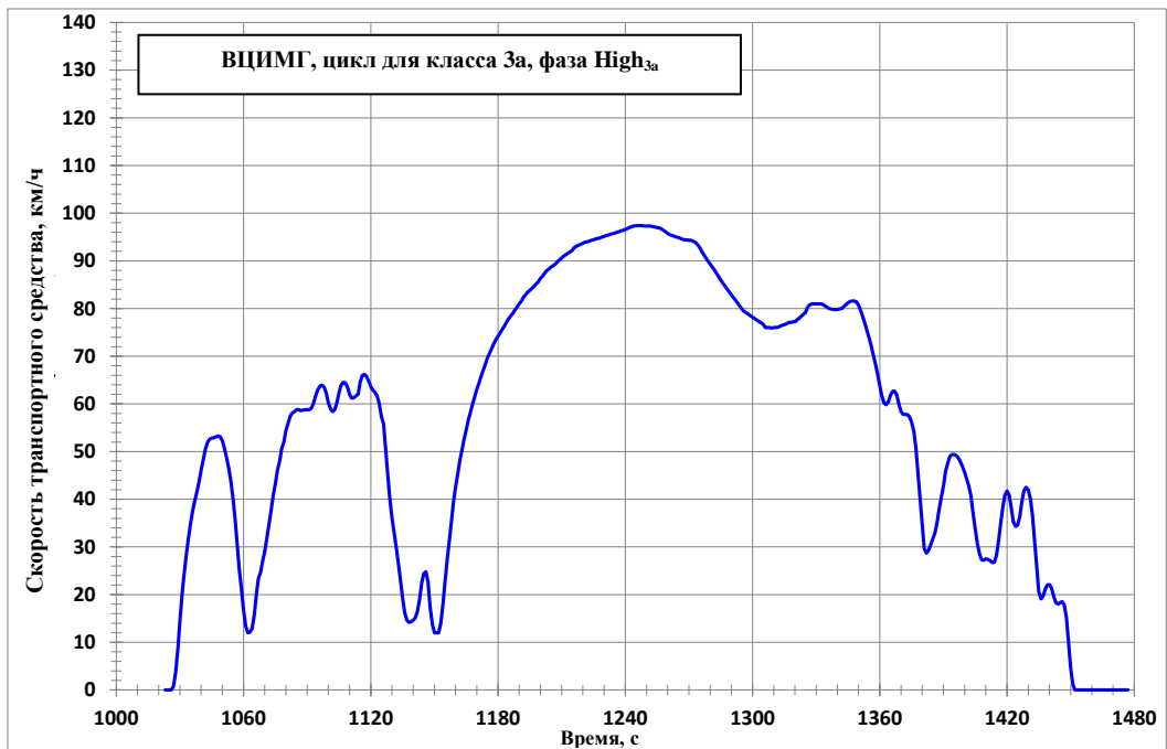
Рис. А1/10 ВЦИМГ, цикл для класса 3a, фаза High 3a
