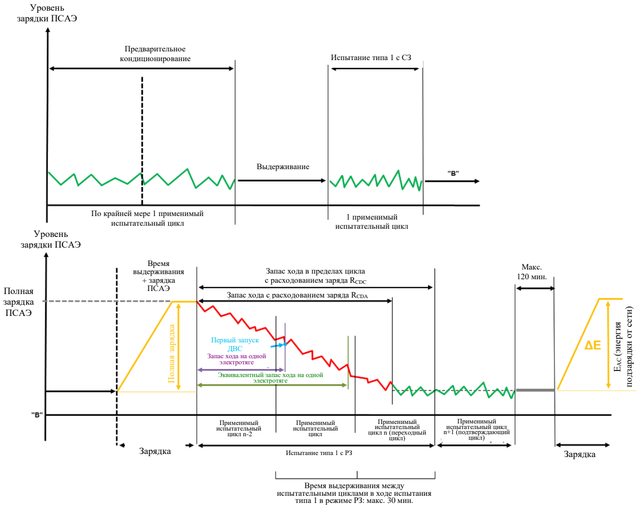
Рис. A8.App1/4 ГЭМ-ВЗУ, испытание типа 1 в режиме сохранения заряда с последующим испытанием типа 1 в режиме расходования заряда
