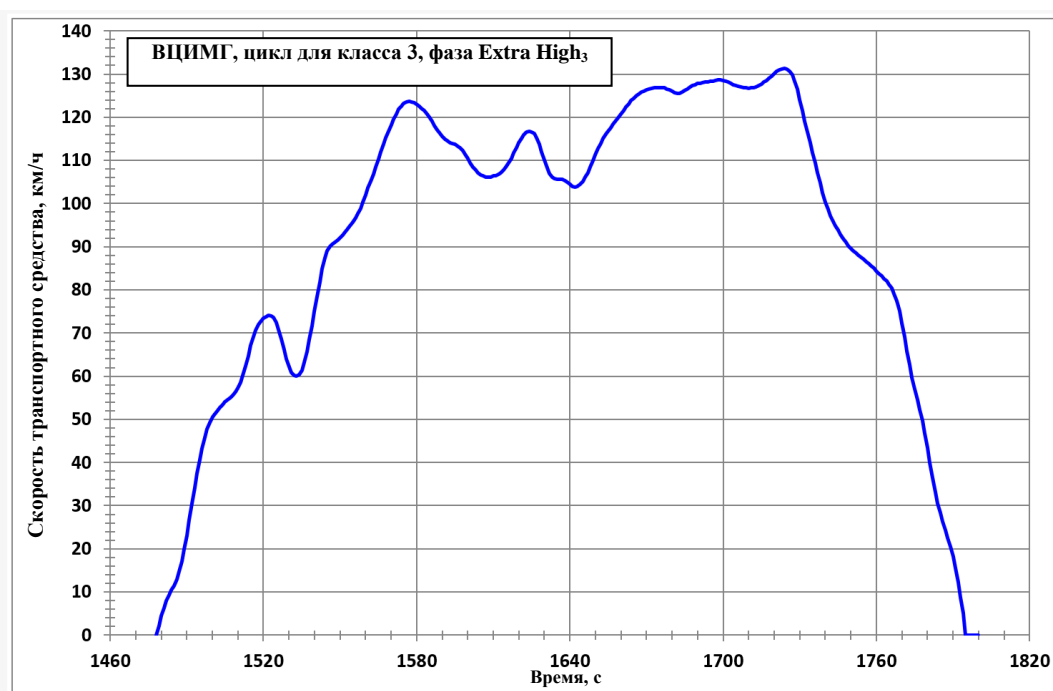
Рис. А1/12 ВЦИМГ, цикл для класса 3, фаза Extra High 3
