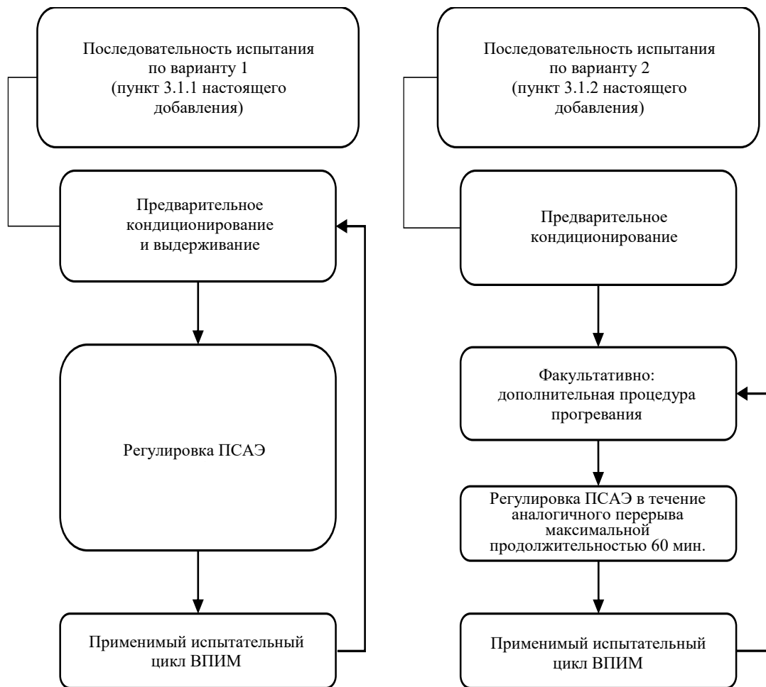
Рис. A8.App2/1 Последовательности испытания ГЭМ-ВЗУ
