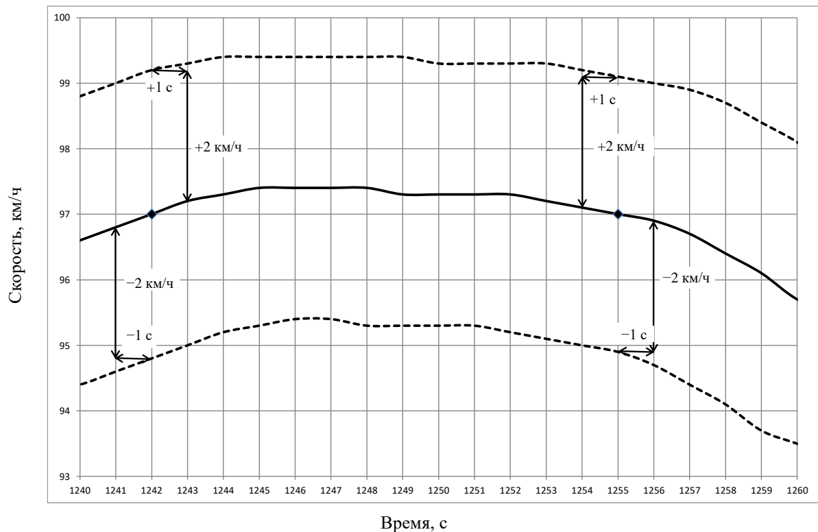
Рис. А6/6 Допустимые отклонения от кривой скорости
