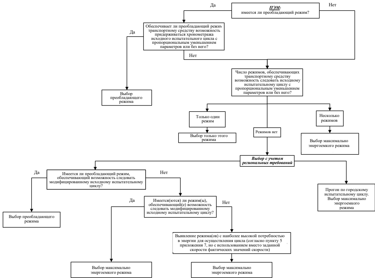
Рис. А8.Аpp6/3 Установка выбираемого водителем режима для ПЭМ
