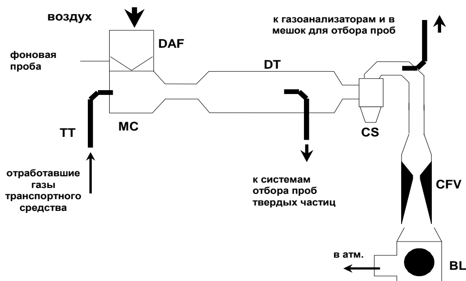
Система разбавления потока с использованием трубки Вентури с критическим расходом
