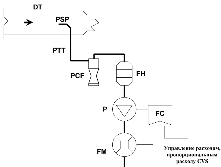
Рис. А4а.Аpp4/12 Система отбора проб взвешенных частиц
