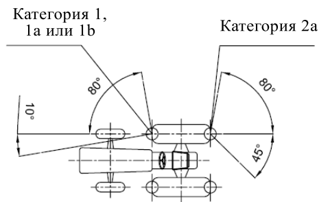
Схема монтажа D
