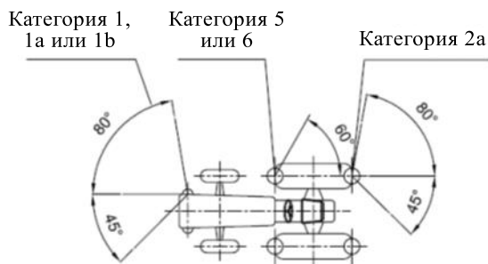
Схема монтажа D
