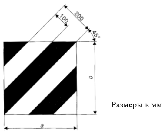
Рис. 2 Сигнальная табличка или сигнальная наклейка
