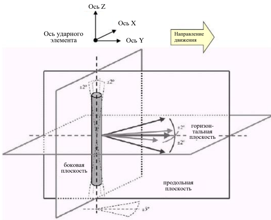
Рис. 3 Допуски на углы первого удара, производимого ударным элементом в виде гибкой модели нижней части ноги
