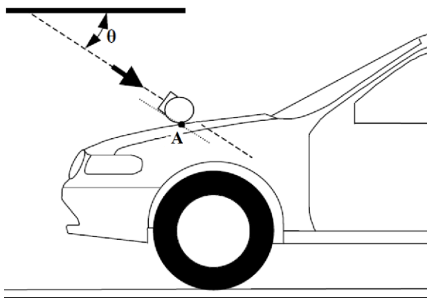
Рис. 8А Измерительная точка в вертикальной продольной плоскости, проходящей через центр тяжести ударного элемента в виде модели головы (см. пункт 2.28.1) 2
