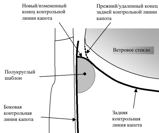
Рис. 4 Определение точки пересечения задней и боковой контрольных линий капота
