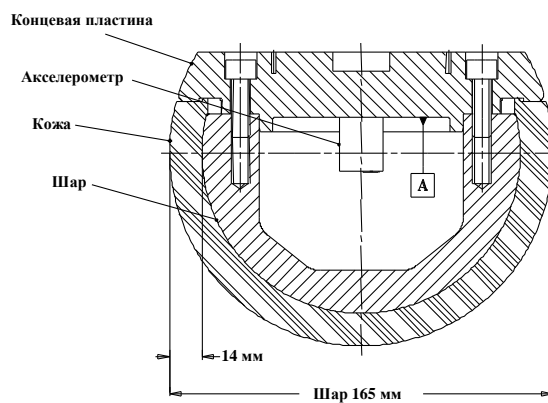
Рис. 5 Ударный элемент в виде модели головы ребенка
