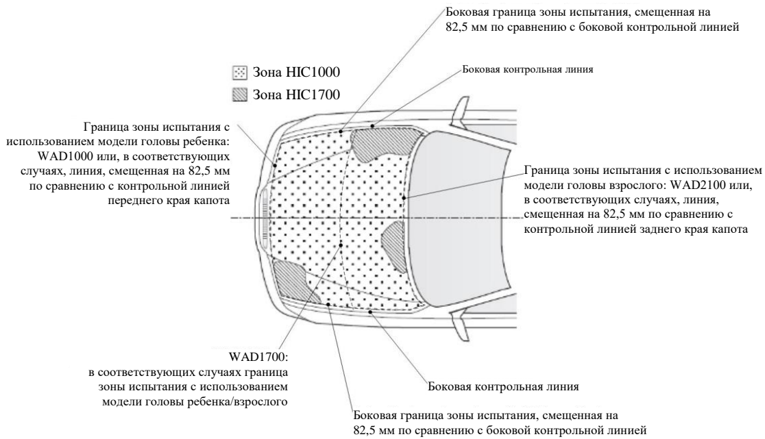
Рис. 5 Пример маркировки зоны НИС1000 и зоны НИС1700
