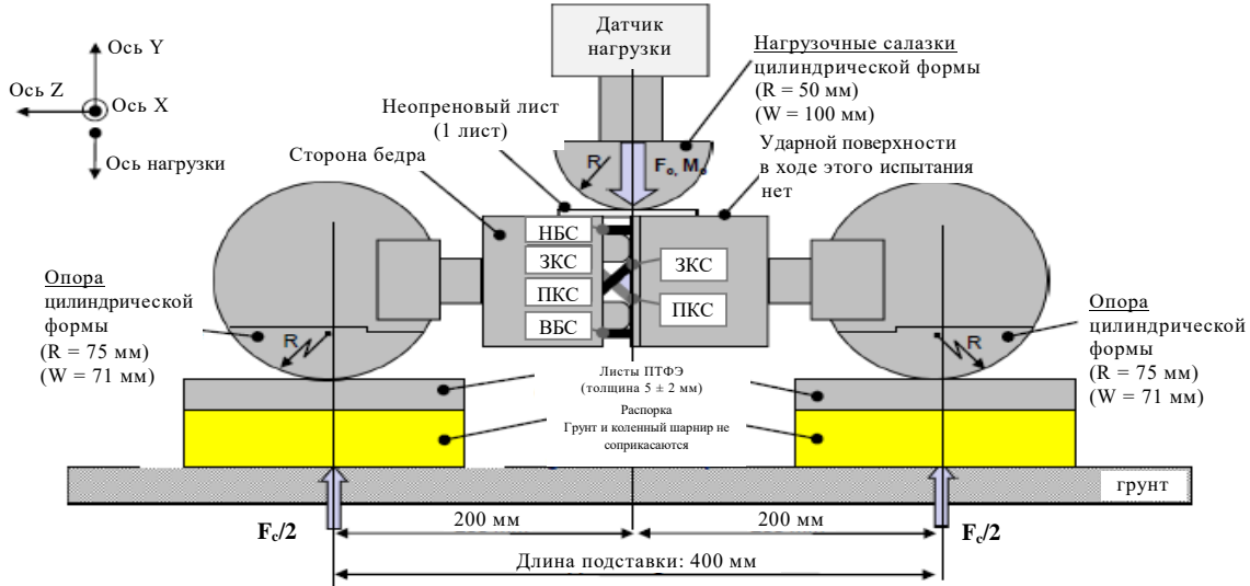
Рис. 5 Ударный элемент в виде гибкой модели нижней части ноги: испытательная установка для проведения испытания коленного шарнира при статических сертификационных испытаниях (см. пункт 1.2.5 настоящего приложения)
