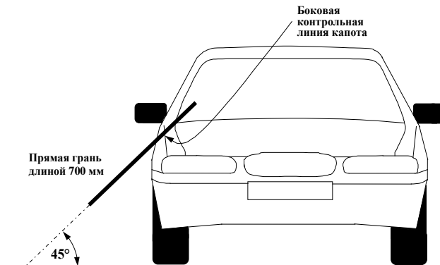
Рис. 9 Боковая контрольная линия
