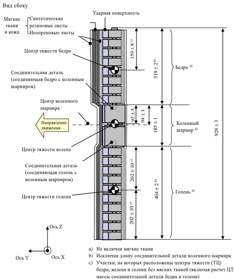
Рис. 1 Ударный элемент в виде гибкой модели нижней части ноги Размеры и участки, на которых расположены центры тяжести бедра, коленного шарнира и голени (вид сбоку)
