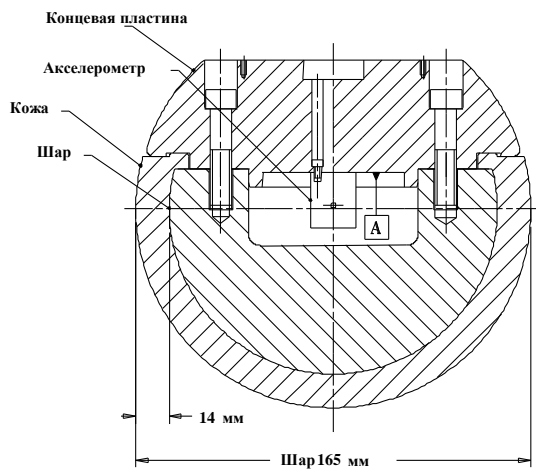
Рис. 6 Ударный элемент в виде модели головы взрослого
