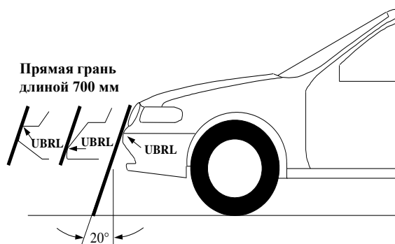
Рис. 10 Контрольная линия верхней части бампера (UBRL)
