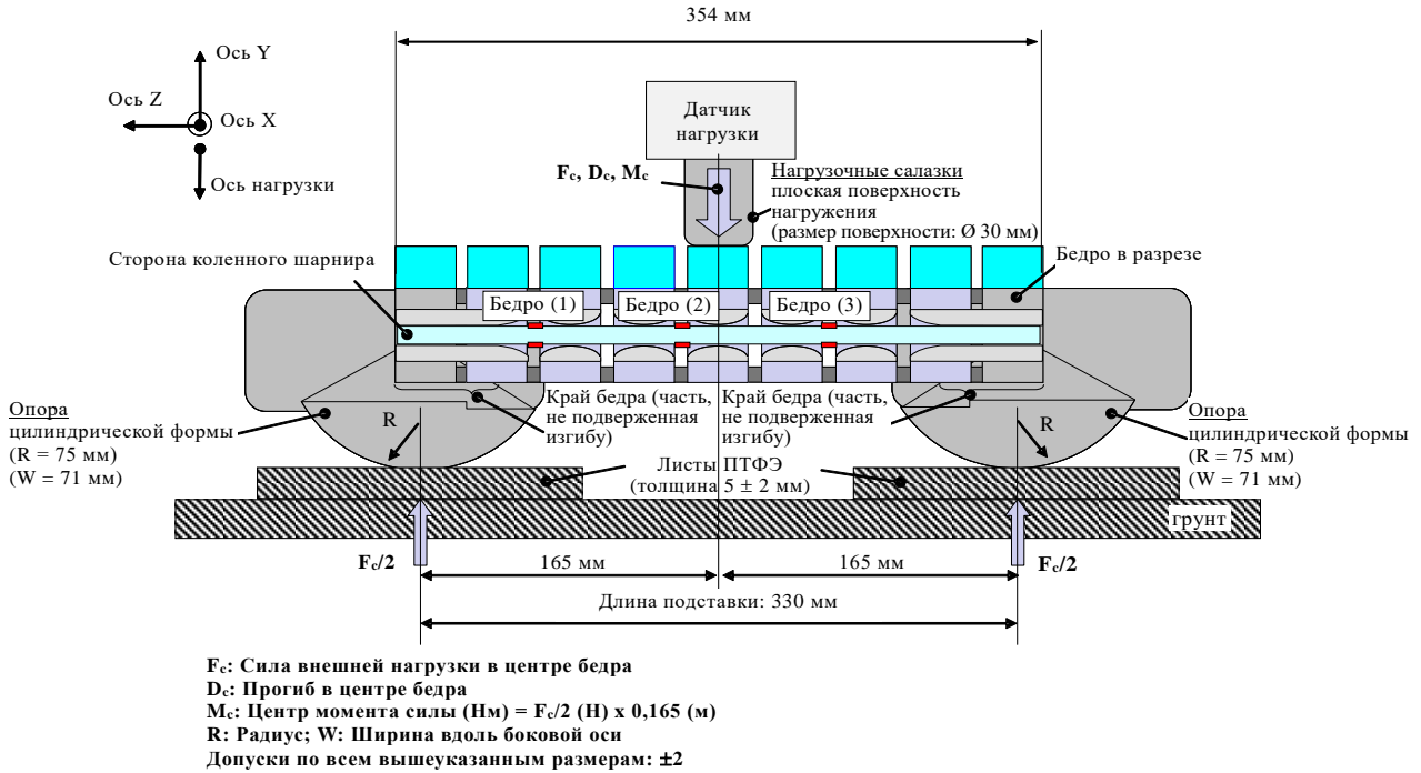
Рис. 3 Ударный элемент в виде гибкой модели нижней части ноги: испытательная установка для проведения испытания бедра при статических сертификационных испытаниях (см. пункт 1.2.4 настоящего приложения)
