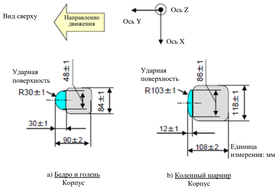
Рис. 2 Ударный элемент в виде гибкой модели нижней части ноги: схема и размеры бедра, голени и колена (вид сверху)
