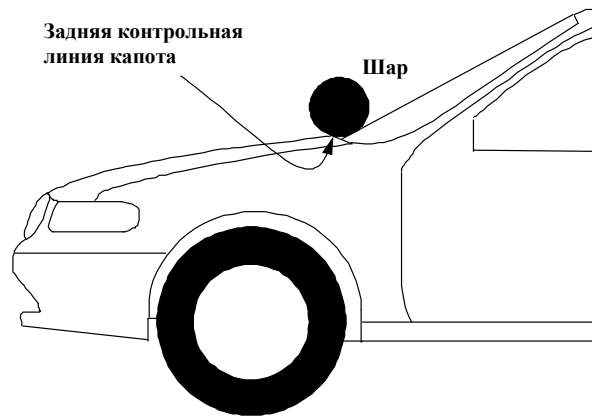
Рис. 2 Задняя контрольная линия капота
