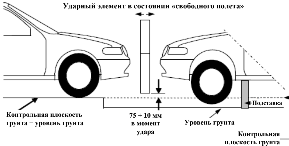
Рис. 4 Испытание бампера с помощью модели нижней части ноги для транспортного средства в сборе в нормальном положении для движения (слева) и для части кузова, установленной на подставке (справа)
