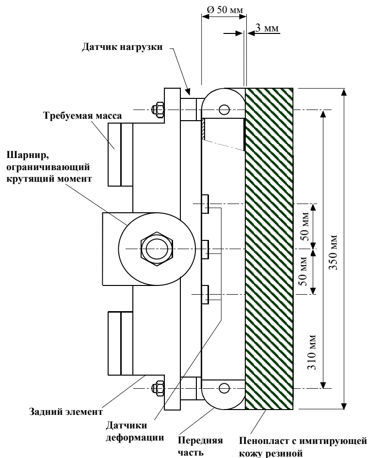
Рис. 4 Ударный элемент в виде модели верхней части ноги
