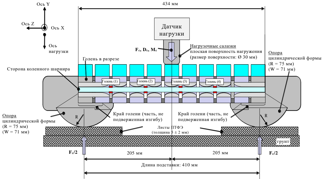
Рис. 4 Ударный элемент в виде гибкой модели нижней части ноги: испытательная установка для проведения испытания голени при статических сертификационных испытаниях (см. пункт 1.2.4 настоящего приложения)
