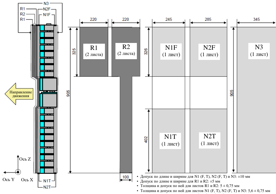
Рис. 2 Ударный элемент в виде гибкой модели ноги: характеристики компрессии элементов, изготовленных с использованием имитирующих мягкие ткани и кожу материалов
