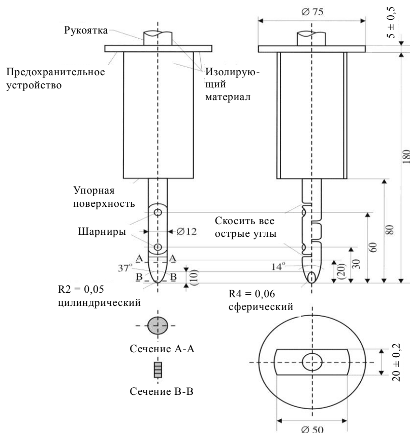
Рис. 1 Шарнирный испытательный штифт
