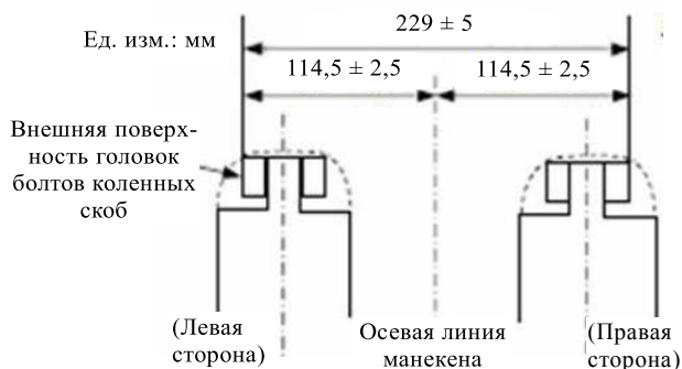
Рис. 2 Первоначальное расстояние между коленями женского манекена «Гибрид III» 5-го процентиля
