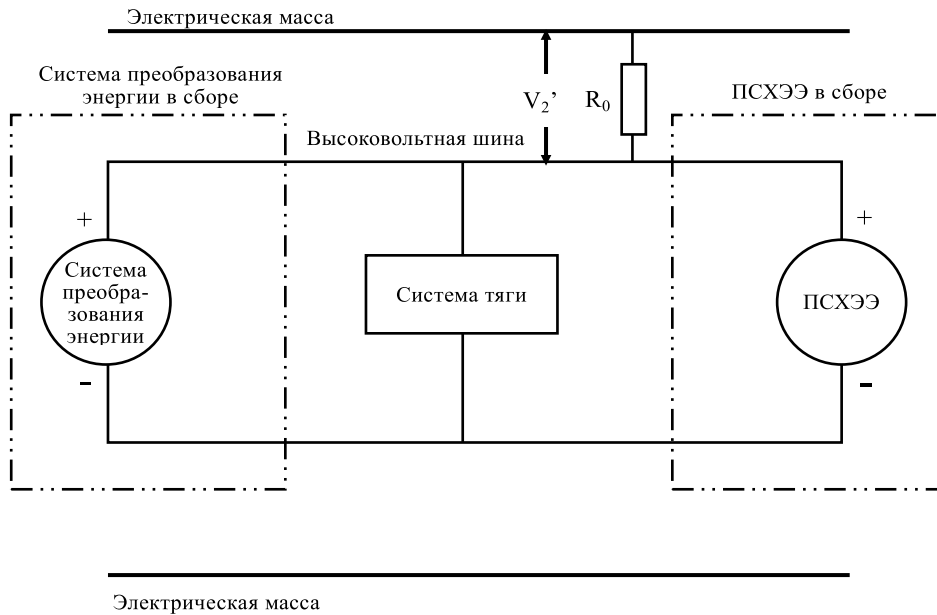
Рис. 4 Измерение V_2'
